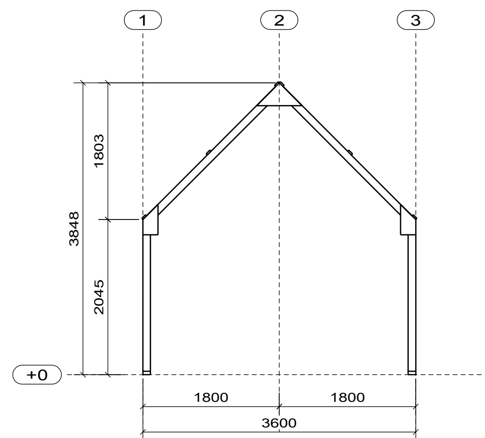
SEKTION MITTRAM
