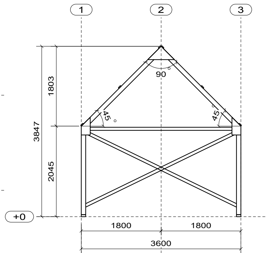
SEKTION GAVELRAM
